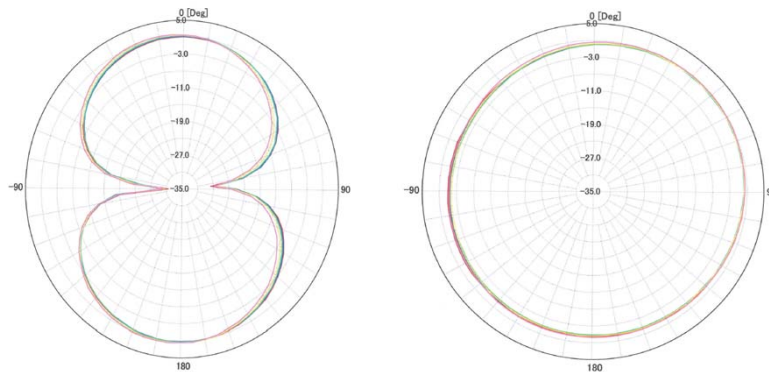
アンテナ放射特性
